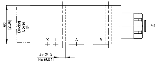
Mit Sekundärdruckbegrenzungsventil (SVA / SVT) With secondary pressure relief valve (SVA / SVT) 带二级溢流阀 (SVA / SVT)
