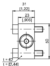
Hubabhängiger Dämpfungsdeckel Typ "D" Hubabhängiger Kerbdämpfungsdeckel Typ "K" Stroke-dependent damping cover with metering grooves type "D" "D" 型行程相关阻尼功能端盖 "K" 型行程相关阻尼功能端盖 · 带沟槽
